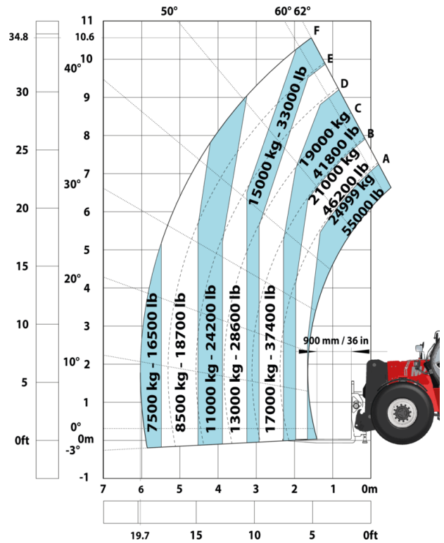
Machine op banden met vorken LC 900 mm
