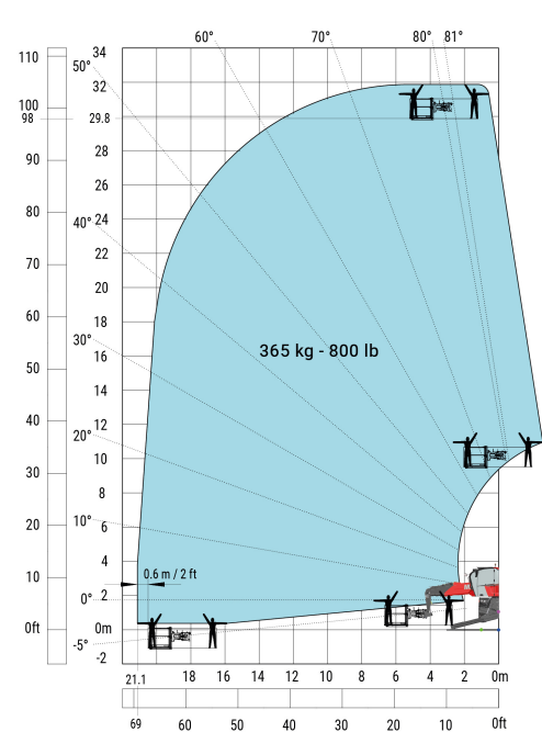
Rotatie op verlaagde stabilisatoren met 365 kg platform
